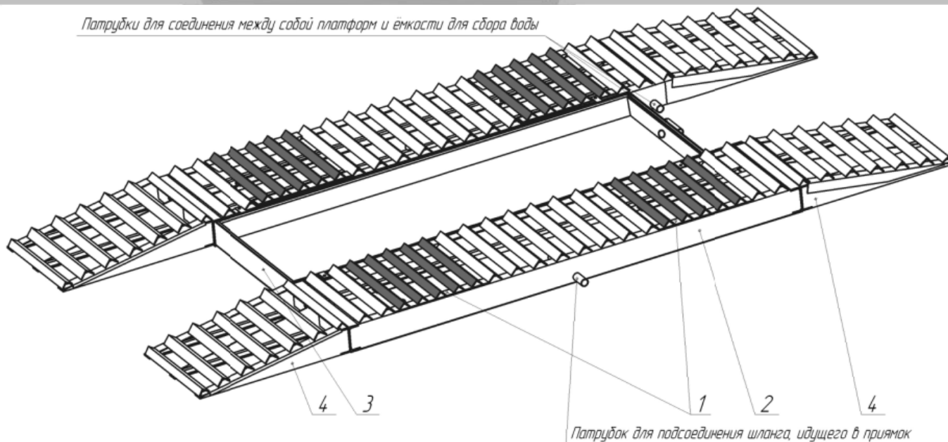
Рис. 2 внешний вид эстакады 3м. В собранном состоянии
